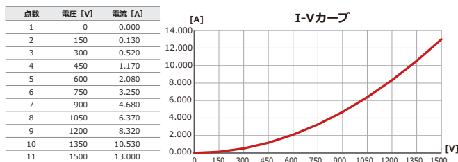
PXZ220K-1500 CCモードの設定例
