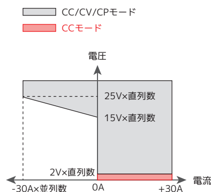
PBWシリーズ低電圧動作範囲
