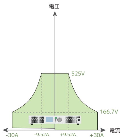
PBW-502H動作範囲
