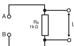
●測定回路網 (ネットワークD 電気用品安全法など)
