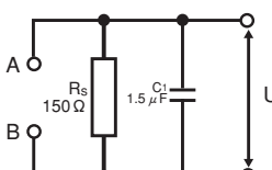
●測定回路網 (ネットワークPCC-2 IEC60598-1)
