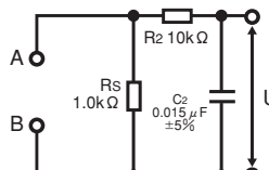
●測定回路網 (ネットワークPCC-1)
