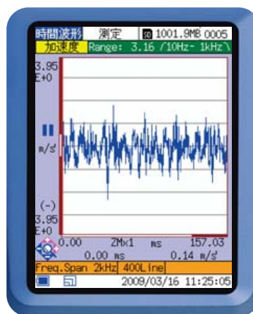
時間波形
