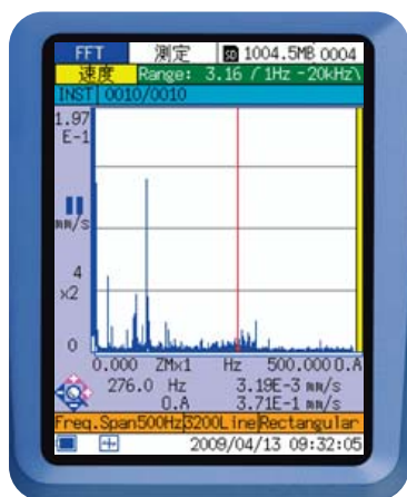
スペクトル
