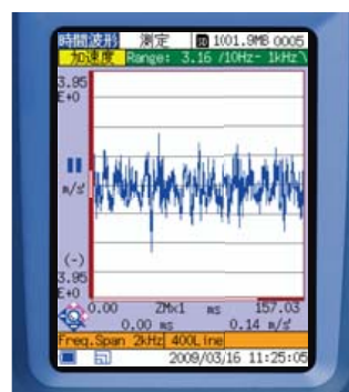
時間波形
