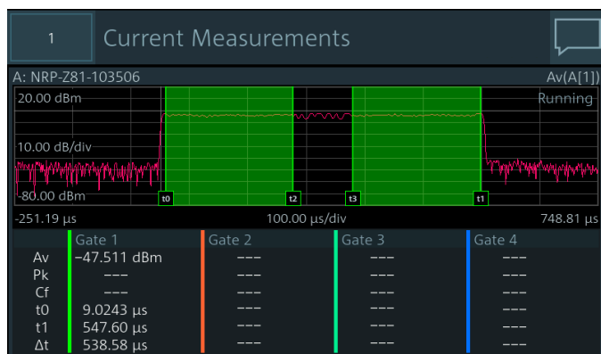
R&S®NRPxxS(N) 3/パス・ダイオード・パワー・センサおよびゲート機能を使用したEDGEパーストのパワーの決定。信号の中心に存在するトレーニングシーケンスを除外します。
