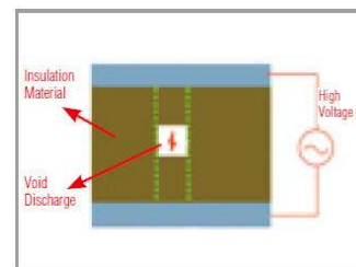
図 9: 空洞放電
