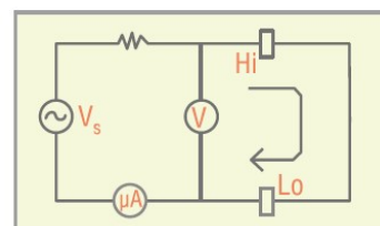
図 3.3：回路短絡時：Cm >> CX
