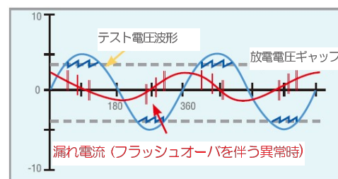
図 2: フラッシュオーバー波形
