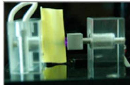
図 1: コロナ放電
