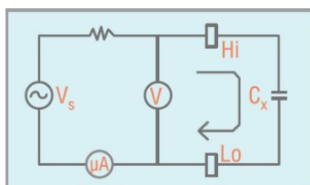
図 3.1：通常状態
