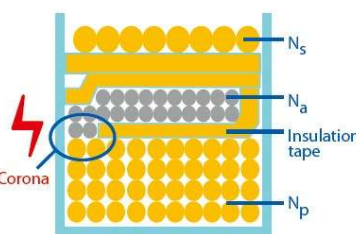
図 7.1: コロナ
