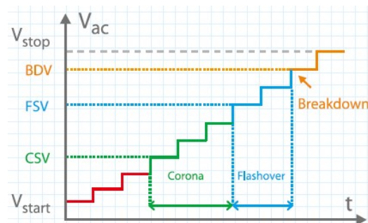
図 4: 放電レベル分析 (DLA)
