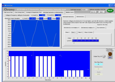
IEC 61000-4-13 高調波と次数間高調波 イミュニティ試験
