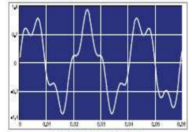
Interharmonics Waveform 次数間高調波波形
