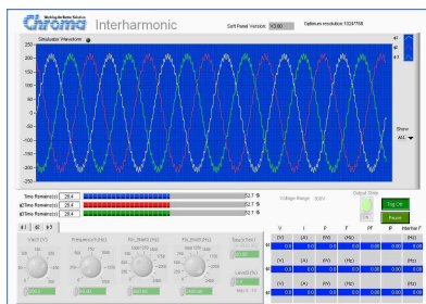
次数間高調波試験画面
