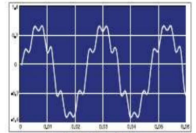
高調波波形
