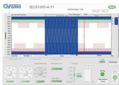
IEC 61000-4-11 電圧ディップ、瞬時停電 イミュニティ試験
