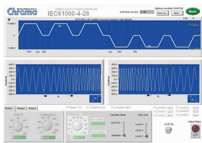
IEC 61000-4-28 電源周波数変動 イミュニティ試験
