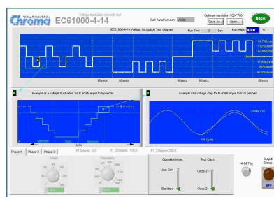
IEC 61000-4-14 電圧変動イミュニティ試験
