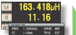
L、Q表示画面(1kHz,CC1mA測定)
