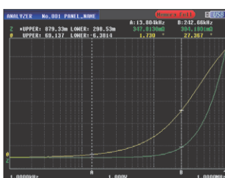
周波数スイープ測定 Z- \theta 測定画面
