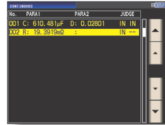
連続測定画面
