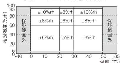
湿度センサ Z2000 使用時精度表
