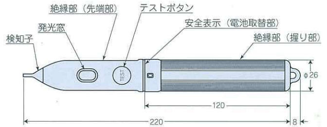
高低圧用検電器 MODEL 5700 (単位mm)
