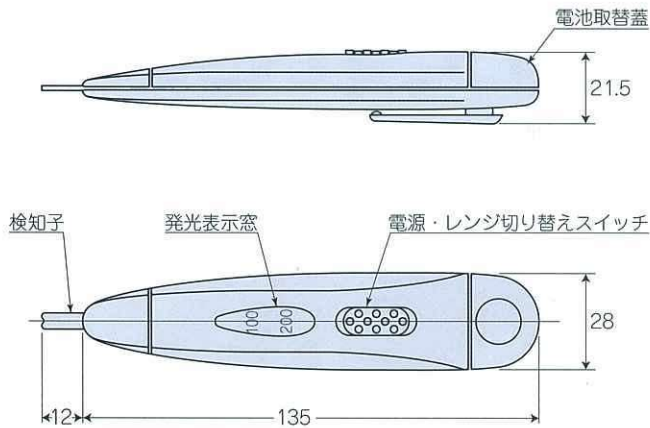
低圧用検電器 MODEL DX-04 (単位mm)
