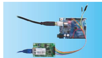
EB-XP011とArduinoとのUART接続例
