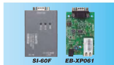
EB-XP061はLAN⇔RS-232CインターフェースコンバータSI-60Fと同じサイズ
