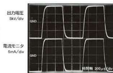
● 定電流モード 1kHz, 10mApk出力 負荷: 抵抗1MΩ
