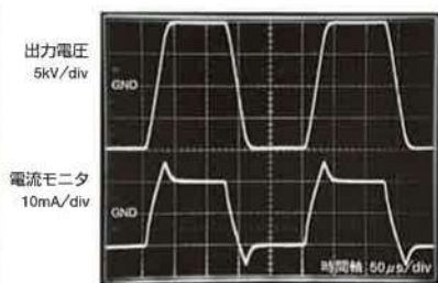
● 定電圧モード 4kHz, 10kVpk出力 負荷: 抵抗1MΩ+ケーブル容量
