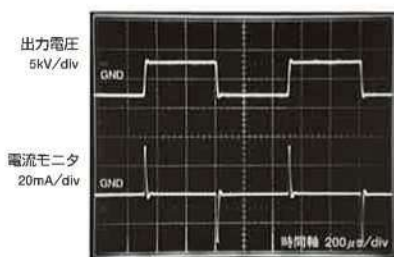
● 定電圧モード 1kHz, 3kVpk出力 負荷: 容量約60pF
