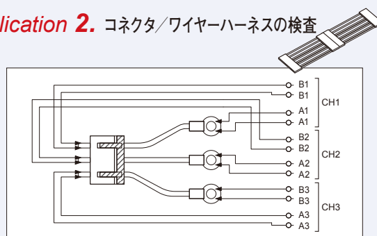
マルチプレクサユニット Z3003 (オプション)
