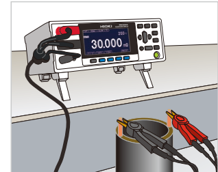
生産ラインで手動測定
