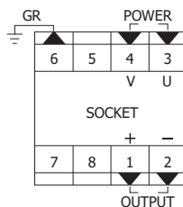
端子配列図
