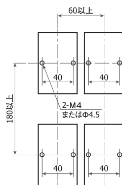
取付寸法図
