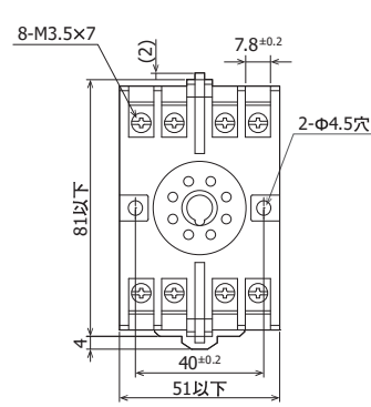
端子台寸法図
