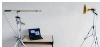
アンテナ ファクタ測定例
