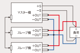
〈並列接続〉
