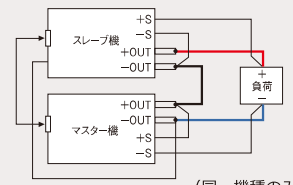
〈直列接続〉
