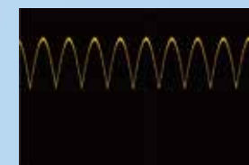
全波整流波形
