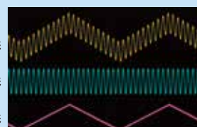
出力波形 加算入力波形 設定波形
