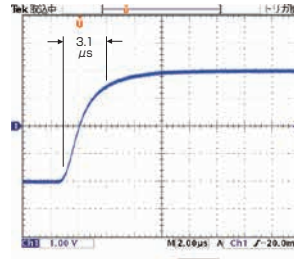
▲ 立上り波形サンプル レスポンス 3.5 μs 設定時
