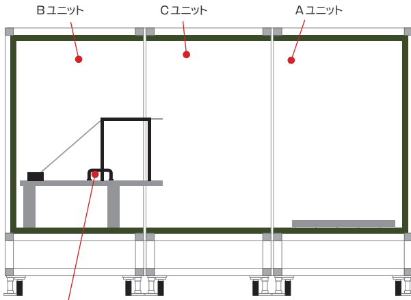
広帯域アンテナ MAN101(オプション)
