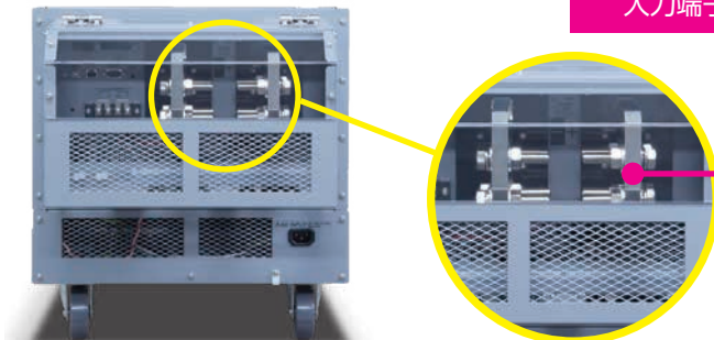
大電流に対応する 入力端子部
