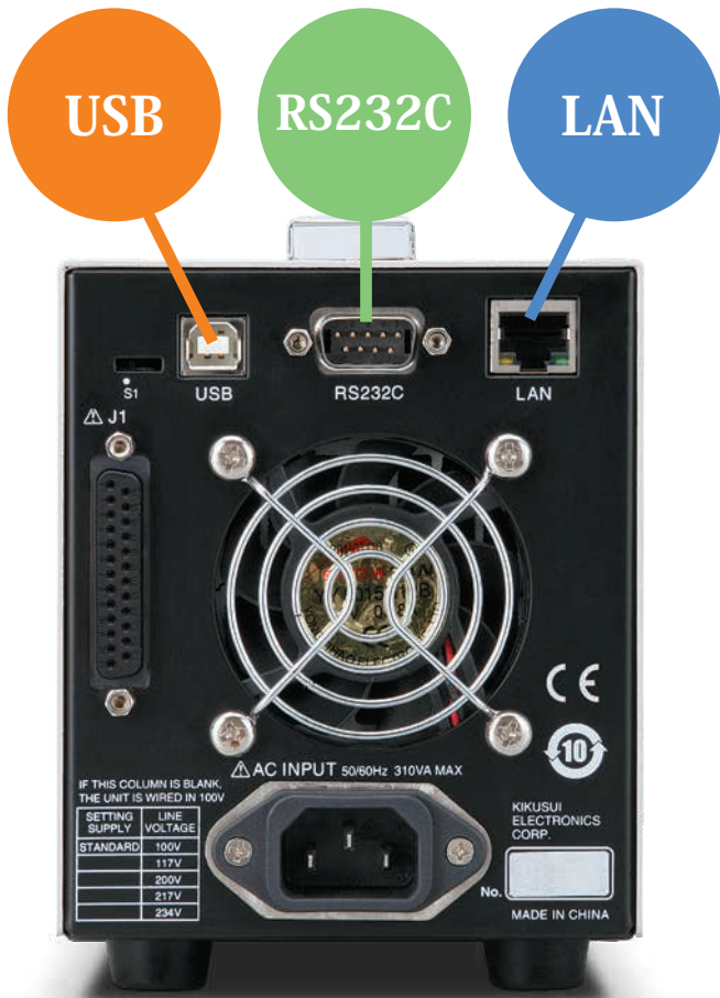
リアパネル
